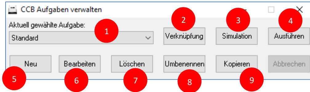
Abbildung 19: Aufgabenverwaltung
