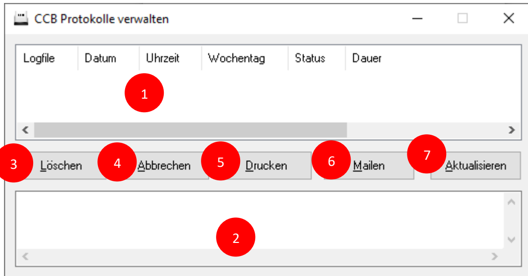
Abbildung 30: Protokollverwaltung
