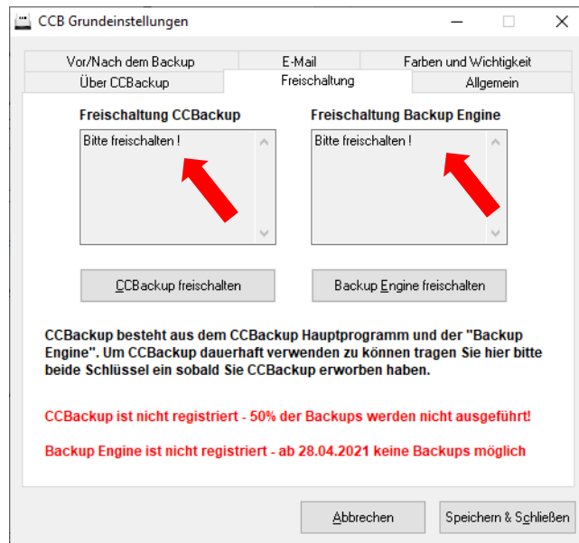
Abbildung 8: Manuelle Freischaltung
