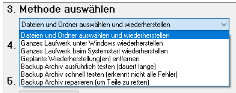
Abbildung 33: Wiederherstellungsmethode
